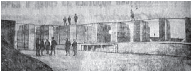
Канал Самур-Дивичи. На снимке: общий вид го-ловного шлюза-регулятора и катастрофического водосброса, законченных строительством на 1-м участке гидротехнических сооружений.
