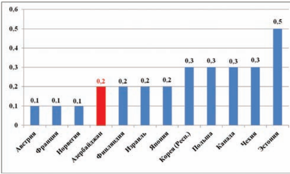
Рисунок 5. Влияние стран ОЭСР на процессы глобального изменения климата: выбросы в атмосферу парниковых газов (кг) при производстве ВВП стоимостью 1 доллар США с учетом ППС. Источник: Всемирный банк, 2019.
